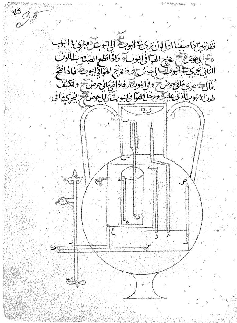
Abb. 120 Konstruktionszeichnung aus dem "Buch der genialen Vorrichtungen" Ms. orient. A 1349, Bl. 35a. 26x19,5 cm (19x13 cm). Banū Mūsā Ibn Šākir: Kitāb al-Ḥiyal .
